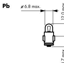
rys.19 Żarówki pomocnicze
