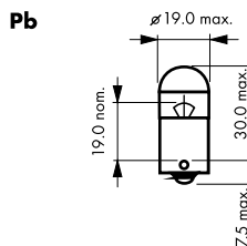
rys.18 Żarówki pomocnicze
