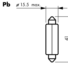
rys.17 Żarówki rurkowe
