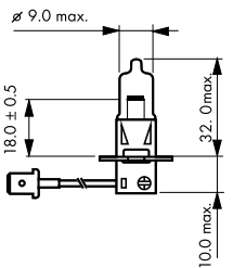
rys.3 Żarówki halogenowe H3
