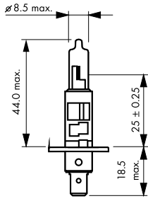
rys.1 Żarówki halogenowe H1
