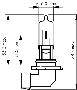
rys.8 Żarówki halogenowe HB3
