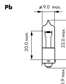
rys.28 Żarówki halogenowe MINI 21 W
