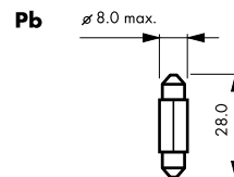
rys.14 Żarówki rurkowe
