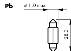
rys.15 Żarówki rurkowe
