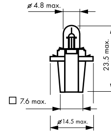
rys.24 Żarówki całoszklane z oprawką
