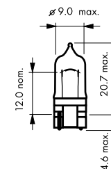
rys.26 Żarówki halogenowe MINI 10 W
