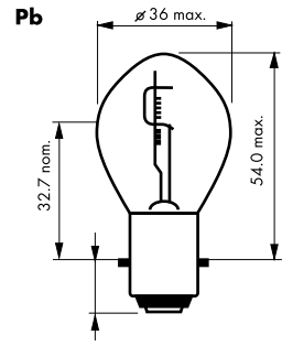
rys.11 Żarówki S1, S2
