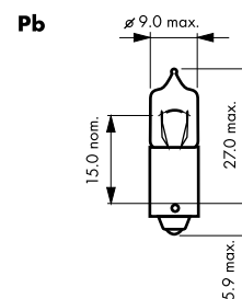
rys.27 Żarówki halogenowe MINI 20 W
