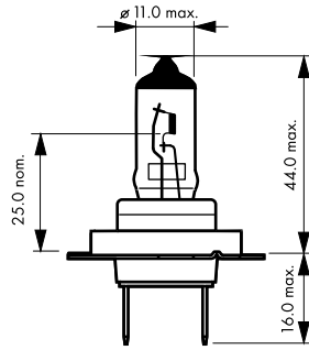
rys.6 Żarówki halogenowe H7
