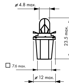
rys.25 Żarówki całoszklane z oprawką
