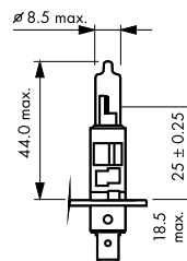
rys.10 Żarówki 12V, 100W, rajdowe
