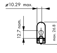
rys.23 Żarówki całoszklane 2W, 3W i 5W
