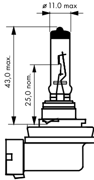
rys.7 Żarówki halogenowe H8
