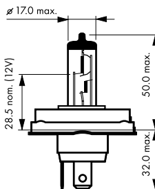
rys.9 Żarówki R2
