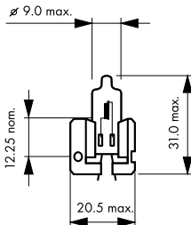
rys.2 Żarówki halogenowe H2
