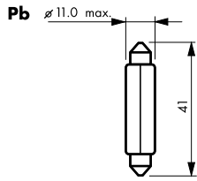
rys.16 Żarówki rurkowe
