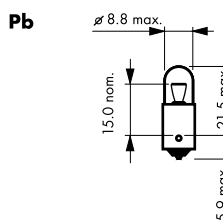
rys.21 Żarówki pomocnicze 6V i 2V 4W
