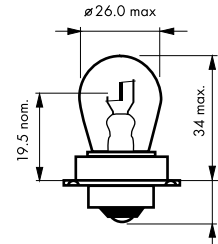
rys.12 Żarówki halogenowe S3
