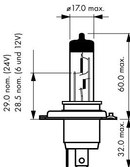
rys.5 Żarówki halogenowe HS1 i H4
