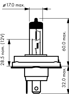
rys.4 Żarówki halogenowe H4
